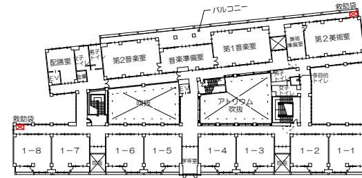
4階平面図
