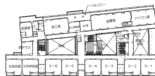
2階平面図
