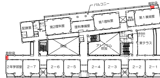
3階平面図
